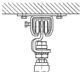
plafondbeugel manchon pour fixation au plafond
