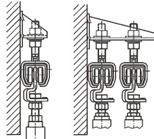
hoek- of dubbele hoekbevestiging fixation d'angle ou double fixation d'angle
