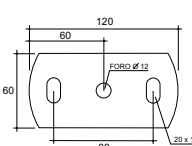
Spessore 8 mm. Art. 15.151.26
