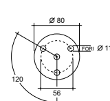
Spessore 6 mm. Art. 15.151.20
