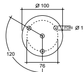
Spessore 8 mm. Art. 15.151.21
