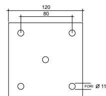
Spessore 8 mm. Art. 15.151.29
