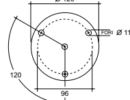
Spessore 8 mm. Art. 15.151.22
