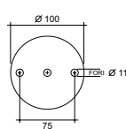
Spessore 8 mm. Art. 15.151.17
