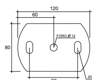
Spessore 8 mm. Art. 15.151.27
