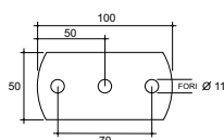
Spessore 8 mm. Art. 15.151.25
