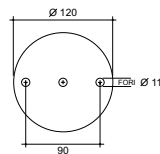
Spessore 8 mm. Art. 15.151.18
