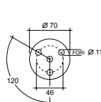
Spessore 6 mm. Art. 15.151.19
