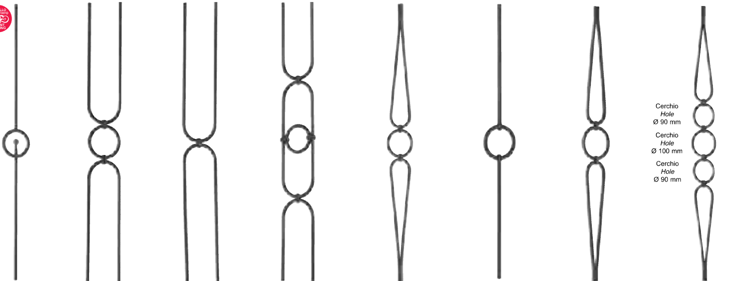
Liscio / Smooth H.950 X L.100 mm. Art. 05.468 Ø 12
