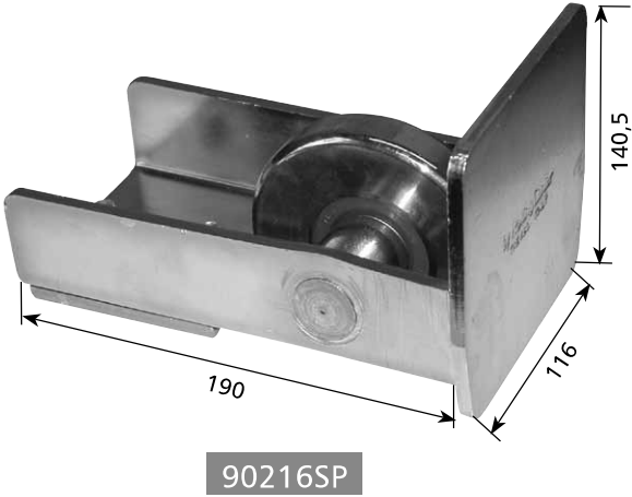
Draagwiel sluitrichting. Roue de support fermeture.
